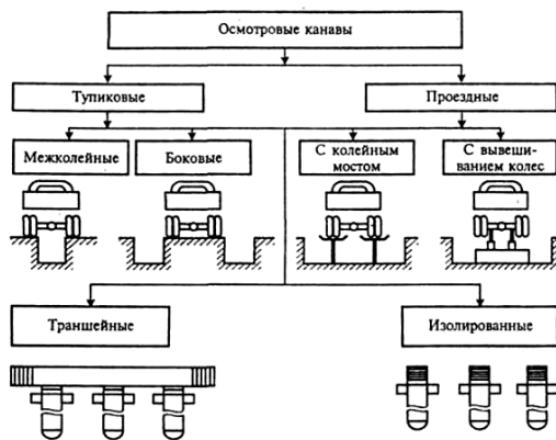
Рис. 72 - Классификация осмотровых канав
