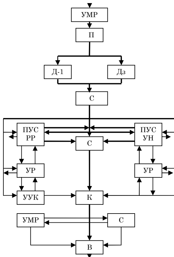
Рис. 33 – Схема технологического процесса обслуживания автомобилей СТО:
