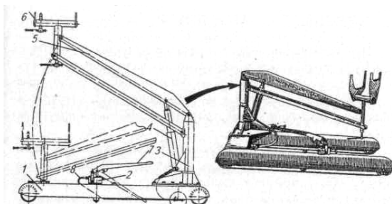
Рис. 90 - Модель - П-208:
