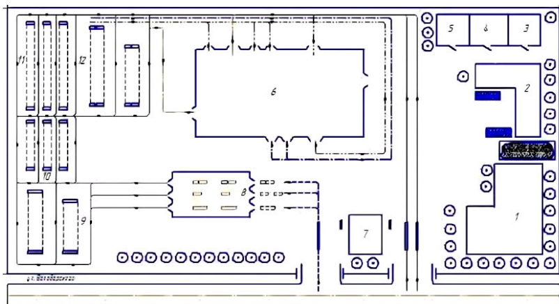
Рис. 43 - Проект АТП на 250 автомобилей:
