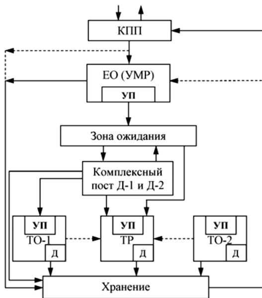
Рис. 31 – Общая схема технологических процессов ТО и ТР для АТП малой мощности
