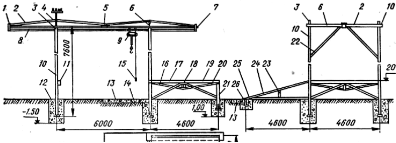
Рис. 47 - Погрузочно-разгрузочная площадка:
