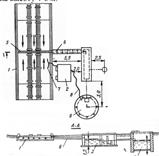
Рис. 46 - Площадка для наружной мойки машин:
