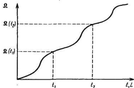
Рис. 52 – Определение нормы расхода запасных частей по ведущей функции потока отказов \Omega(t)
