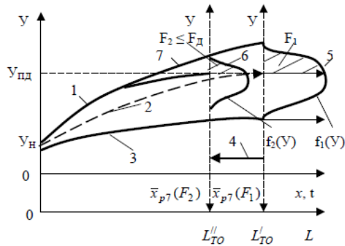
Рис. 18 – Определение периодичности L_{TO} по допустимому значению и изменению параметра технического состояния
