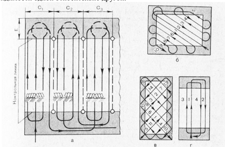
Рис. 39 - Способы движения тракторных агрегатов:
