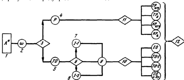
Рис. 25 - Схема формирования структуры системы ТО и ремонта автомобилей:
