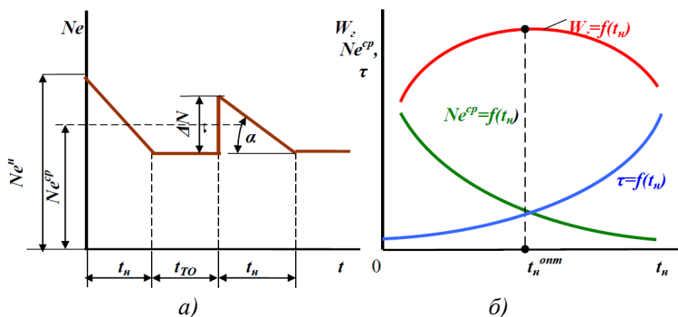
Рис. 23 - Изменение мощности (а), производительности и параметров, на нее влияющих (б), в зависимости от срока работы машины ( tn ) и продолжительности ТО ( t_{TO} )
