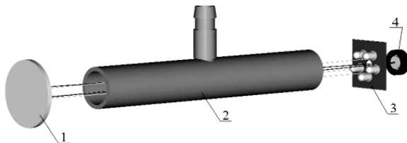
Рис. 95 - Оптическая схема дымомера:
