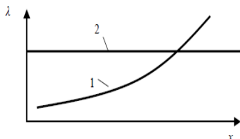
Рис. 10 – Изменение интенсивности постепенных (1) и внезапных (2) отказов
