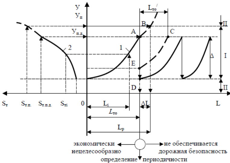
Рис. 13 - Схема изменения и восстановления технического состояния
