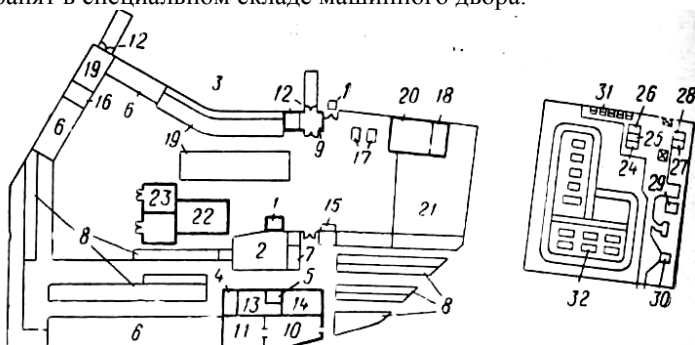
Рис. 50 - Материально-техническая база технического обслуживания машинно-тракторного типовой проект 816-33:
