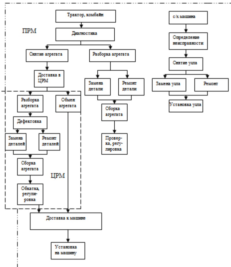
Рис. 35 – Схема технологического процесса ремонта в полевых условиях
