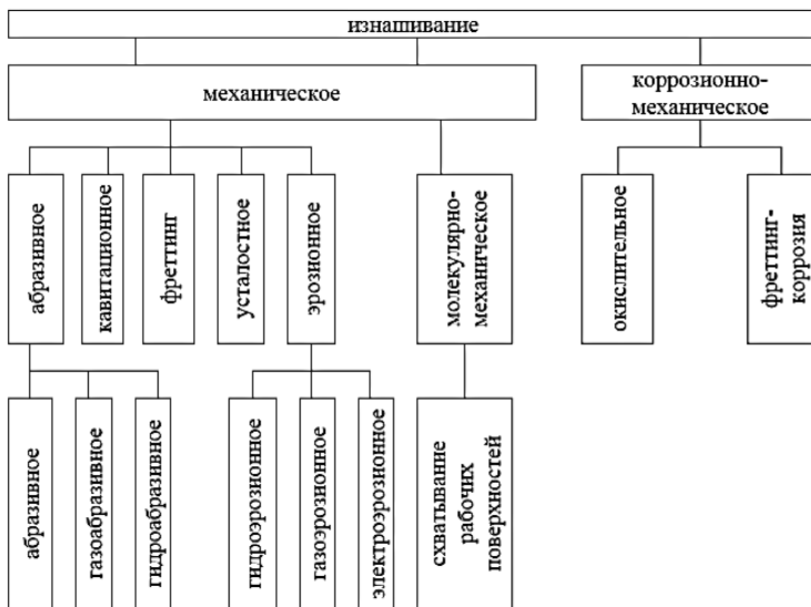
Рис. 4 - Виды изнашивания
