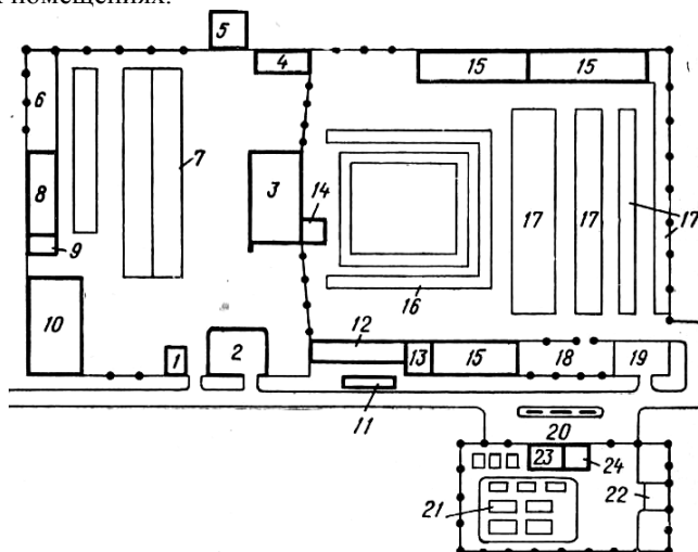
Рис. 49 - Производственно-техническая база технического обслуживания машинно-тракторного парка на 50 тракторов:
