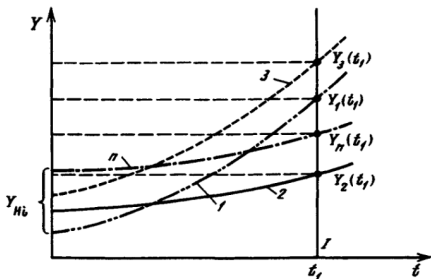
Рис. 7 - график формирования случайного процесса:
