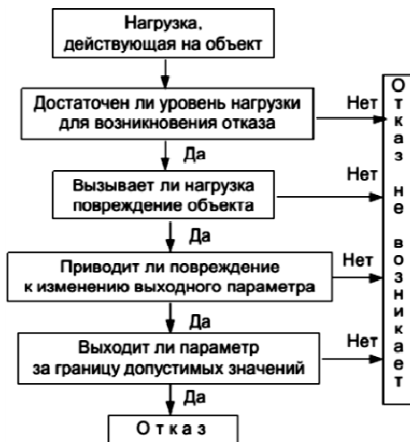
Рис. 1 – Схема возникновения отказа
