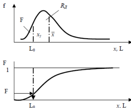
Рис. 16 – Определение периодичности ТО по допустимому уровню безотказности
