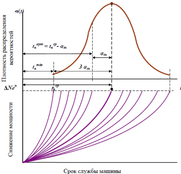
Рис. 24 - Схема определения периодичности технического обслуживания машины
