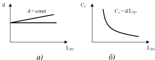
Рис. 20 - Изменение d и C_1 в зависимости от периодичности
