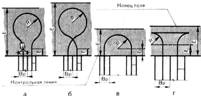
Рис. 41 - Схемы поворотов тракторных агрегатов на концах гона:
