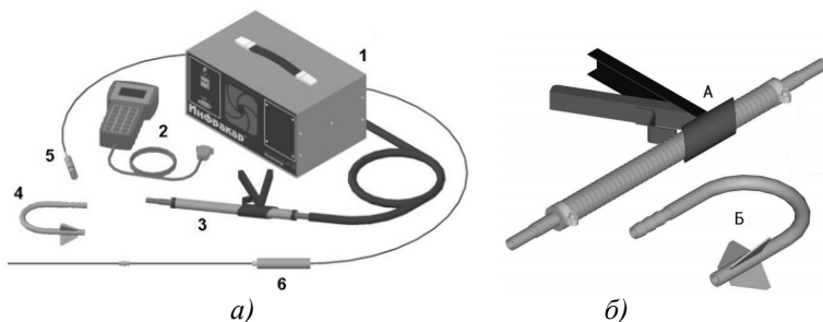
Рис.96 - Дымомер Инфракар Д:
