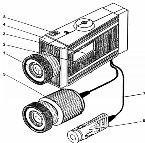
Рис. 93 - Внешний вид прибора ЛЮКС МС-2:
