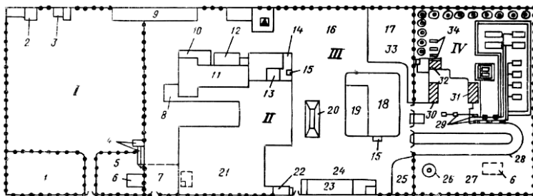
Рис. 48 - Производственно-техническая база технического обслуживания и ремонта машинно-тракторного парка:
