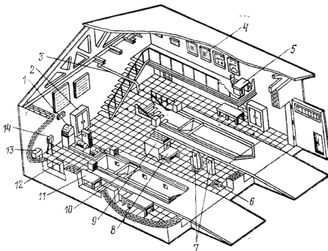
Рис. 45 - Пункт технического обслуживания
