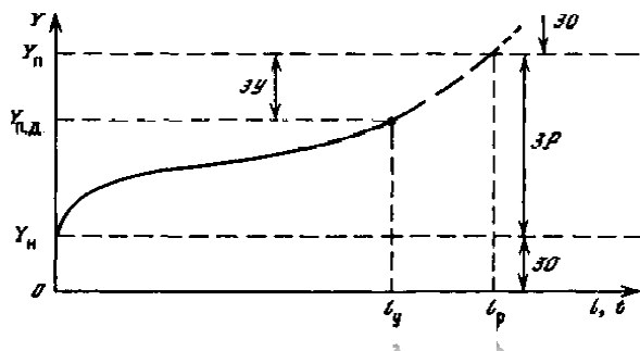
Рис. 3 – Схема изменения параметров технического состояния:
