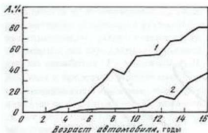
Рис. 6 - Тенденции изменения местной (1) и общей (2) коррозии при старении легковых автомобилей:
