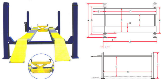
Рис. 79 - Модель П-4.5ПГ
