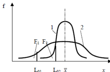
Рис. 17 – Влияние вариации на оптимальную периодичность
