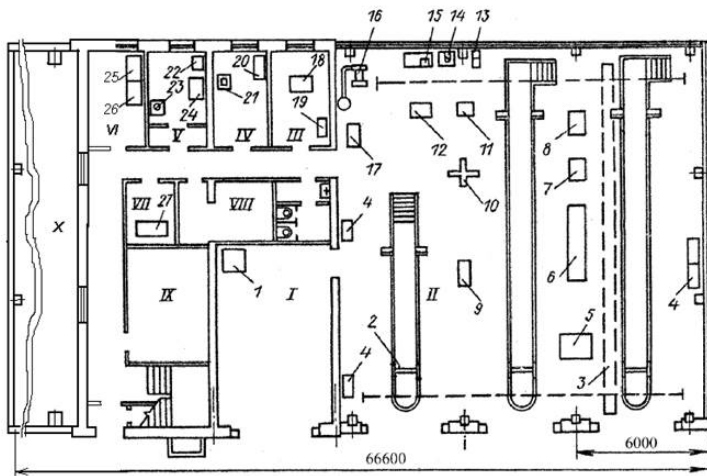
Рис. 44 - План размещения производственных участков и технологического оборудования гаража с техническим профилактором для обслуживания 60 автомобилей:
