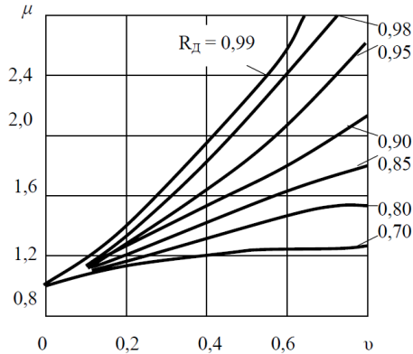
Рис. 19 – Влияние коэффициента вариации \nu на коэффициент максимально допустимой интенсивности \mu
