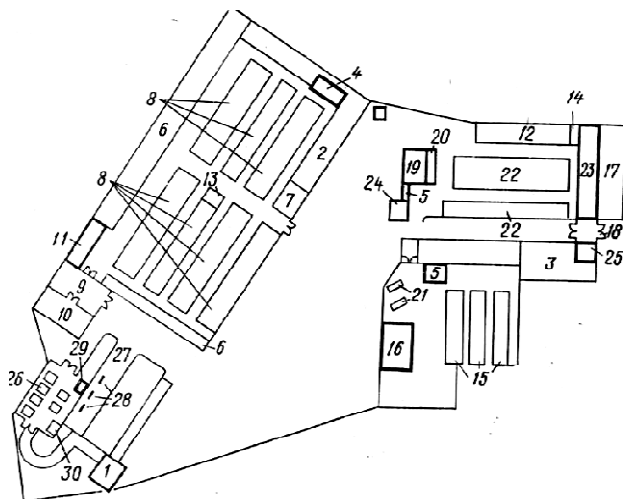
Рис. 51 - Производственно-техническая база технического обслуживания машинно-тракторного парка на 100 тракторов:
