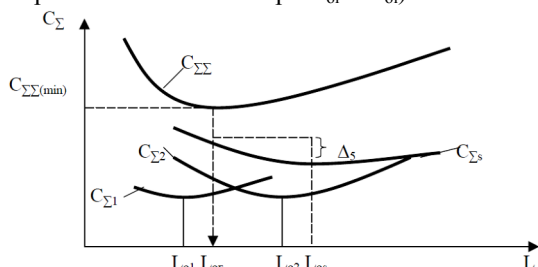
Рис. 27 – Определение групповой периодичности ТО технико-экономическим методом:
