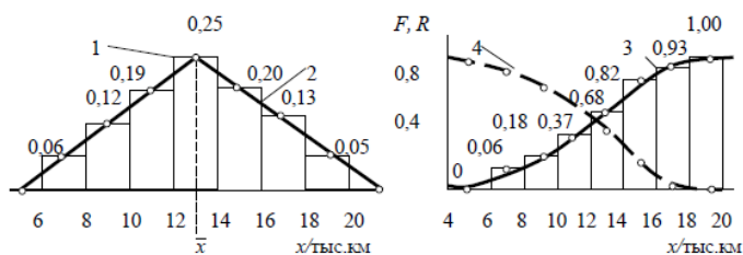
Рис. 11 – Графическое изображение случайной величины:
