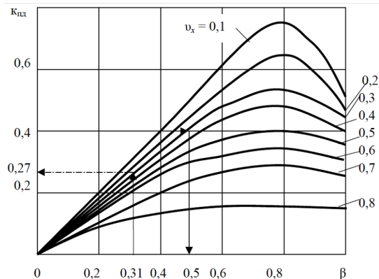
Рис. 28 – Оценка рациональности профилактических воздействий при заданной периодичности
