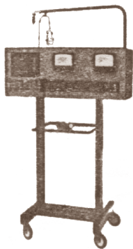
Рис. 68 - АНАЛИЗАТОР К 518-03
