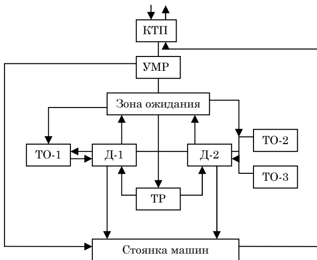
Рис. 34 – Схема технологического процесса ТО и ТР машинно-тракторного парка
