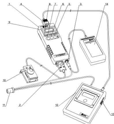
Рис. 97 - Внешний вид прибора модификации «Эффект-02»:
