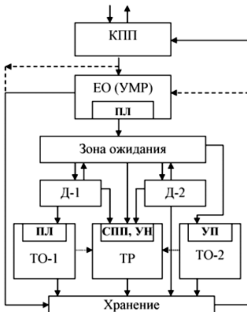
Рис. 32 - Общая схема технологических процессов ТО, Д, ТР для АТП средней мощности:
