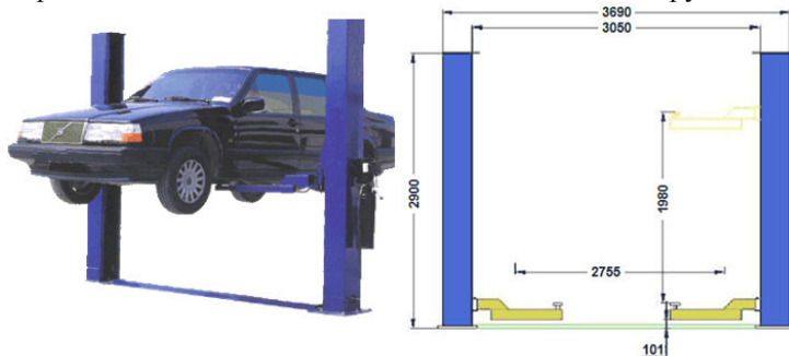
Рис. 74 – Подъемник П-3.2Г
