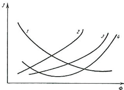
Рис.5 - Зависимость интенсивности изнашивания J от обобщенных безразмерных факторов:
