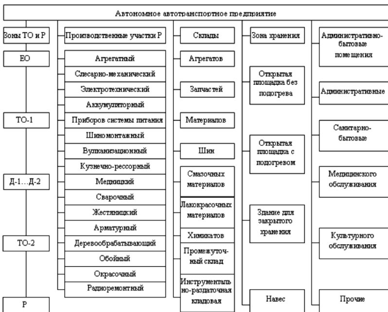
Рис. 42 - Структура производственно-технической базы автономного автотранспортного предприятия
