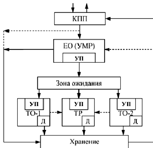
Рис. 30 – Общая схема технологического процесса ТО и ТР для АТП особо малой мощности:
