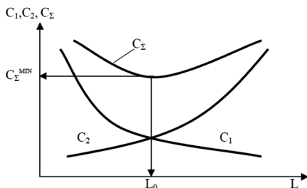
Рис. 22 – Изменение удельных затрат в зависимости от периодичности ТО
